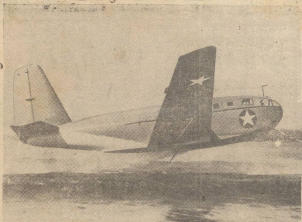
DESILISADORES ANFIBIOS — O tipo de desilizador autônomo desenvolvido pela Marinha dos Estados Unidos para ser empregado em ataques de invasão ao território ocupado pelo "eixo". É construído de madeira laminada, pode transportar vários soldados perfeitamente equipados e outro material bélico, oferecendo a grande vantagem de uma amerisagem silenciosa nas praias inimigas. (Foto da Inter-Americana).
