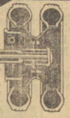
Eixo traseiro inteiramente flutuante. Engrenagem em espiral, com pinhão montado entre rolamentos.
