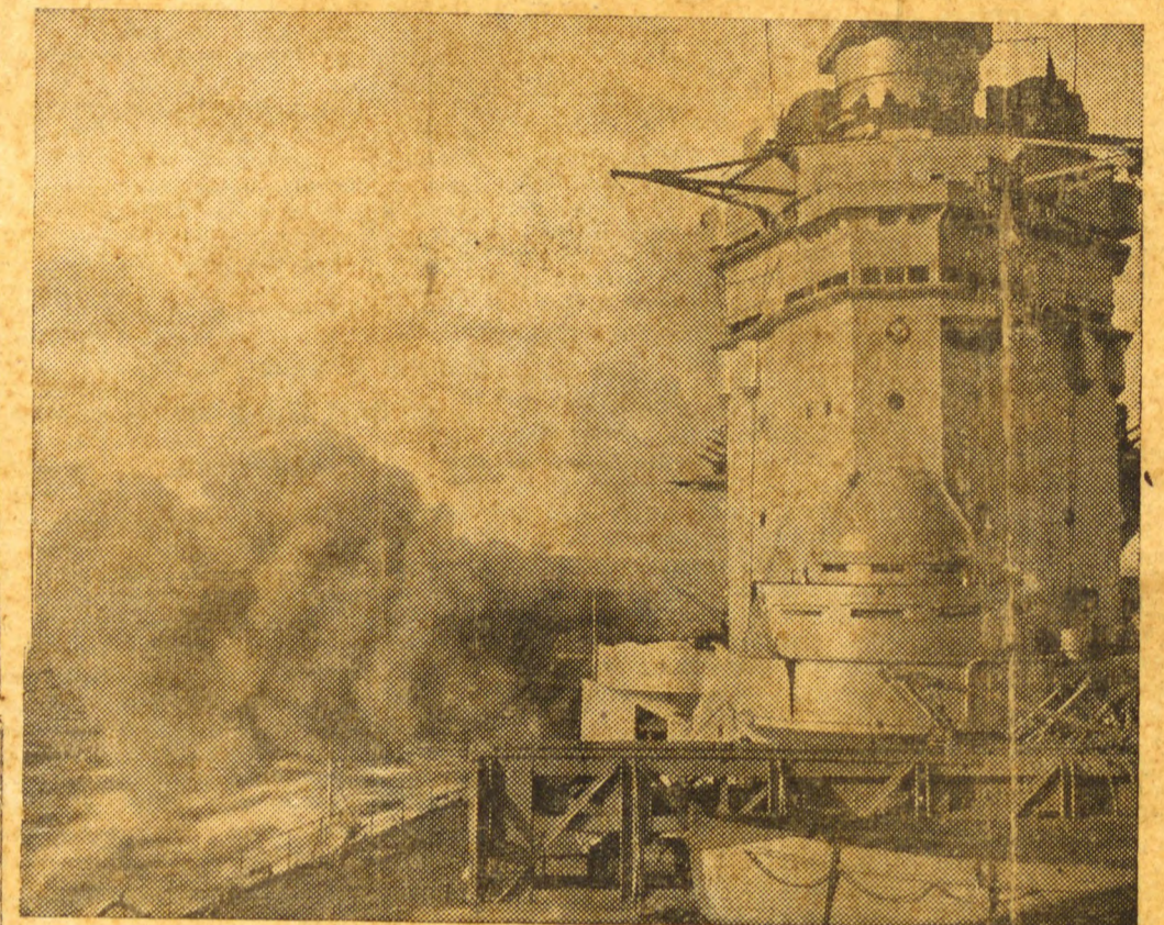
A FORTALEZA MARITIMA — Poder e força são expressos em todas as linhas deste magistoso vaso de guerra da Marinha Real Britânica. Enquanto o navegador todos os marinheiros acham-se em seus postos, com balas nos seus canhões e metralhadoras prontas para disparar logo que o inimigo é avistado. O navio da fotografia está atirando com o segundo armamento, que são canhões de 6 pol. — (British News Service)
