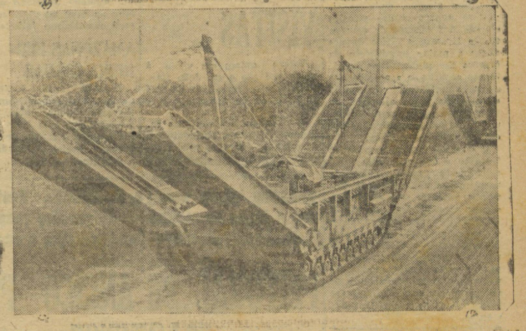
A PONTE DE AUTO-PROPULSÃO DO EXERCITO BRITANICO O novo método de lançamento de pontes ideado pelo engenheiro britânico para a travessia de pequenos cursos d'agua, fossos e valas, foi de grande utilidade na campanha contra a Alemanha na Europa e contra os japoneses na Birmania. A fotografia mostra um “tank” especial lança-ponte movendo-se ao longo de uma estrada, na Italia. As rampas podem ser vistas claramente. (Foto B. N. S.)
