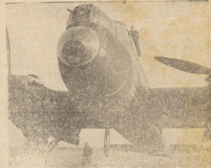
O NOVO BOMBARDEIRO GIGANTE DA RAF — O "AVRO MANCHESTER". — O novo bi-motor da RAF, o "Avro Manchester", que tem estado em serviço desde ha varios mezes, durante os quais já tomou parte em varios raids contra Berlim e outras grandes cidades alemãs, transporta uma grande carga de explosivo e dispõe de ottimo armamento defensivo, incluindo 2 metralhadoras na torre da frente, 4 na ré e outras 2 na torre dorsal do centro da fuselagem. O "Manchester" tem uma envergadura de ponta a ponta de 42 metros, um pouco mais de 90 pés, isto é, quasi exatamente 30 metros. A gravura acima nos mostra a prôa do grande aparelho, vendo-se a cabine do bombardador e as duas metralhadoras da torre fronteira. BRITISH NEVVS SERVICE.
