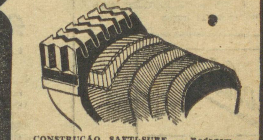
CONSTRUÇÃO SAFETY-SURE —Rodagem e carcassa indissoluvelmente soldadas num só conjunto de resistência extra. Criação FIRESTONE.
