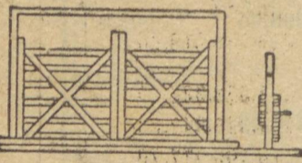
MODELO 3535 BALANÇA PARA PESAR GADO Construção em ferro forjado e aço especial temperado
