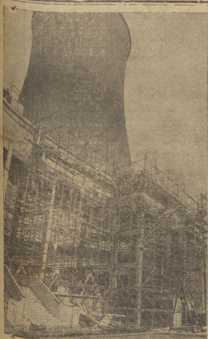
I.B.7 — MAIS ELETRICIDADE NA INGLATERRA. Durante a guerra, as dificuldades impediram a construção de usinas elétricas na Inglaterra. Mas agora foi iniciada a construção de uma série de instalações com as quais se espera compensar as deficiências até 1950. Esta torre de refrigeração é maior já construída. Tem uma altura de 320 pés e um diâmetro de 226.
